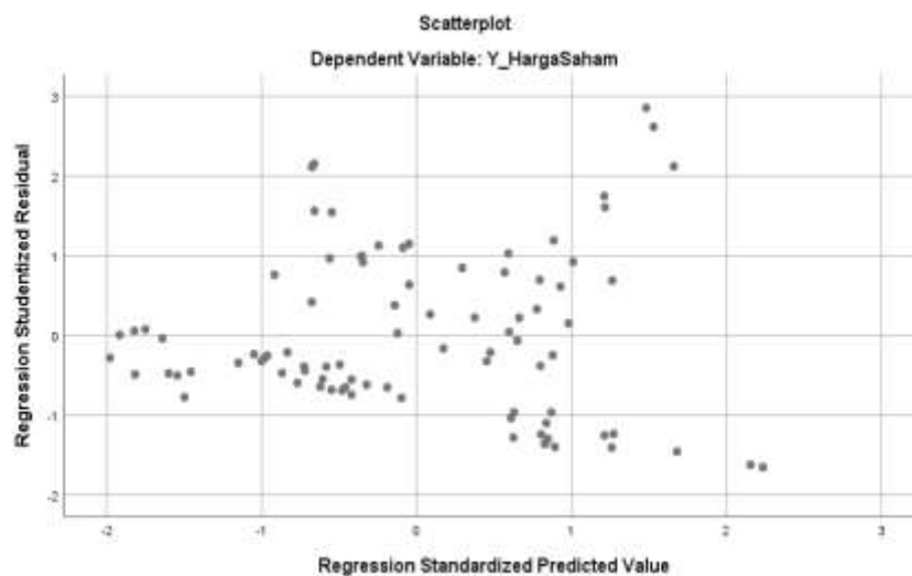
Gambar 1 Uji Heterokedastisitas
