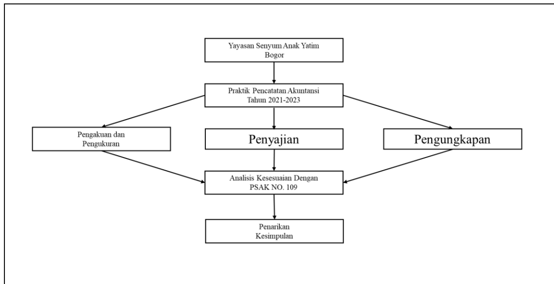
Gambar 1. Kerangka Berpikir
